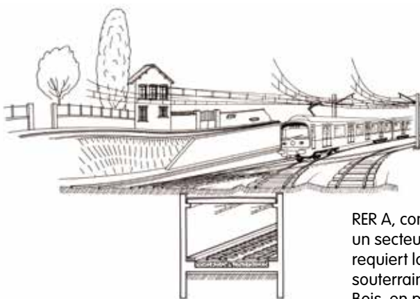
Plan détaillant la construction du souterrain pour le futur RER A à Fontenay-sous-Bois. Vers 1975 (©AD94)
